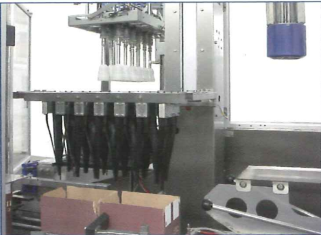
Imbuti centratori per cartoni con alveari preinseriti Centering funnels for cartons with pre-made partitions Entonnoirs de centrage pour cartons avec ruche préintroduites
